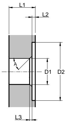
Ferramenta especial para rebaixar e chanfrar
